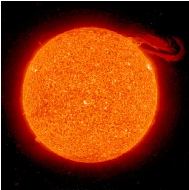
Le Soleil tel que vu dans l'ultraviolet « lointain » (UVC) image en « fausses couleurs »).
